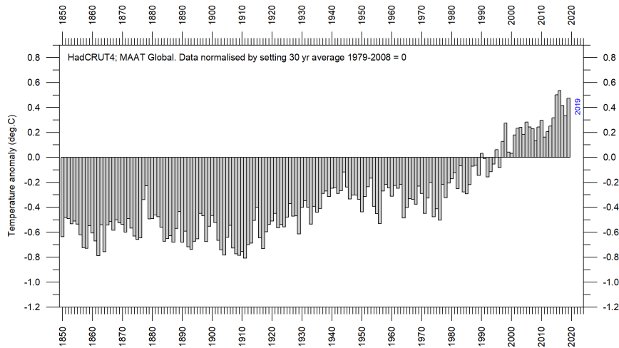
(a) HadCRUT4
