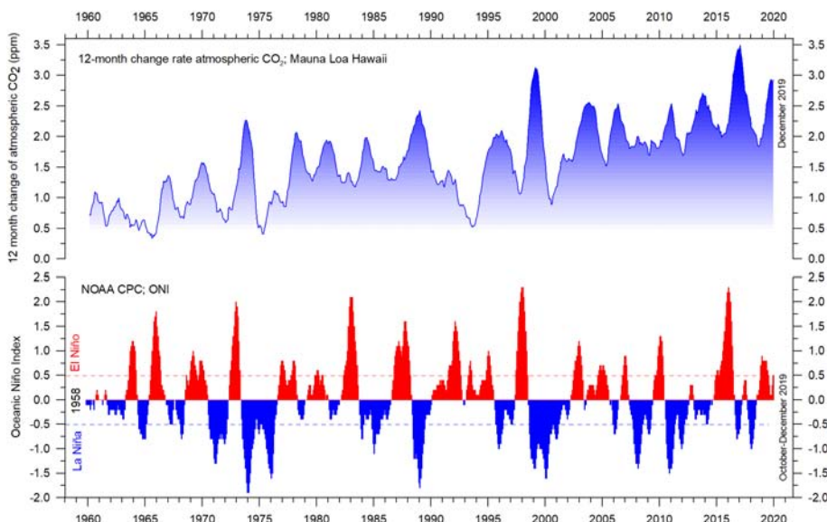
Figure 16: CO 2 and El Niño.
