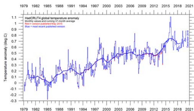
(a) HadCRUT4
